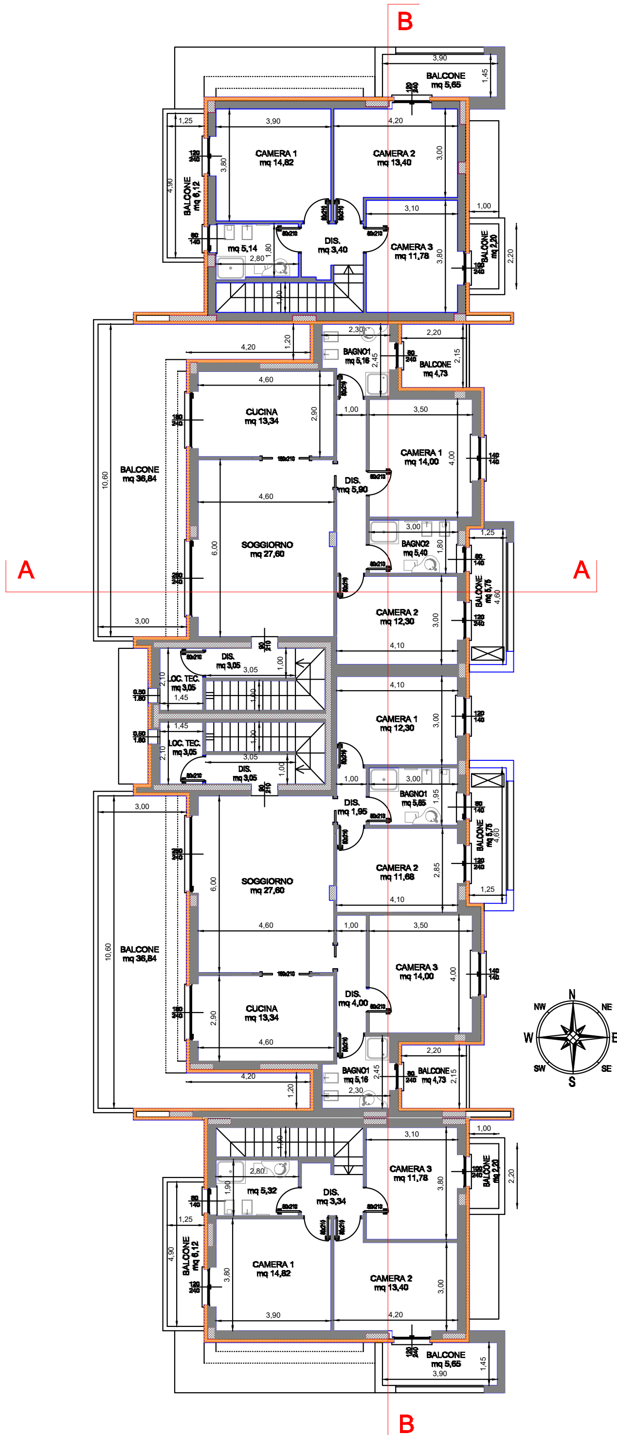
PIANTA PIANO PRIMO scala 1:100
