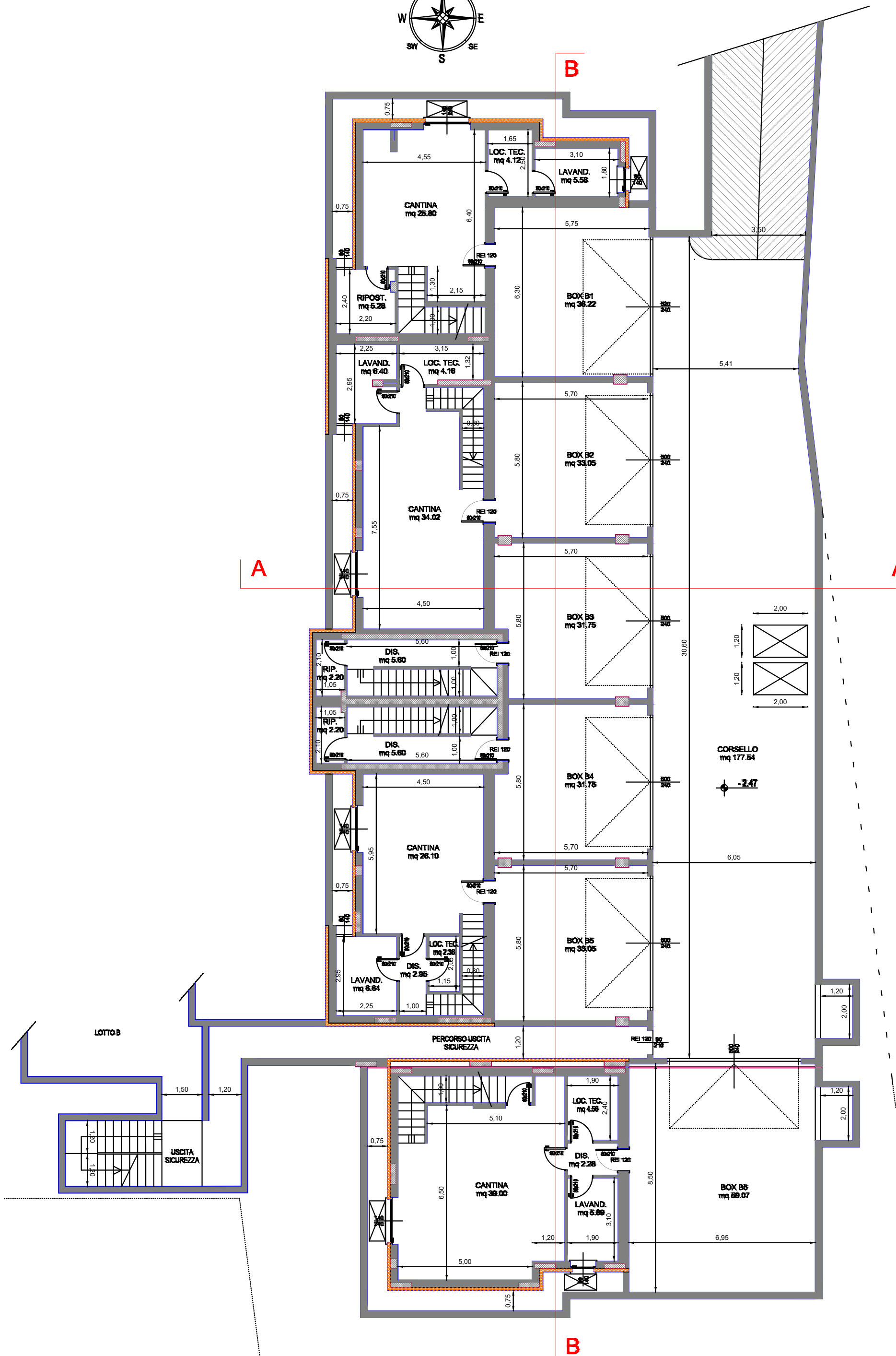
PIANTA PIANO INTERRATO scala 1:100
